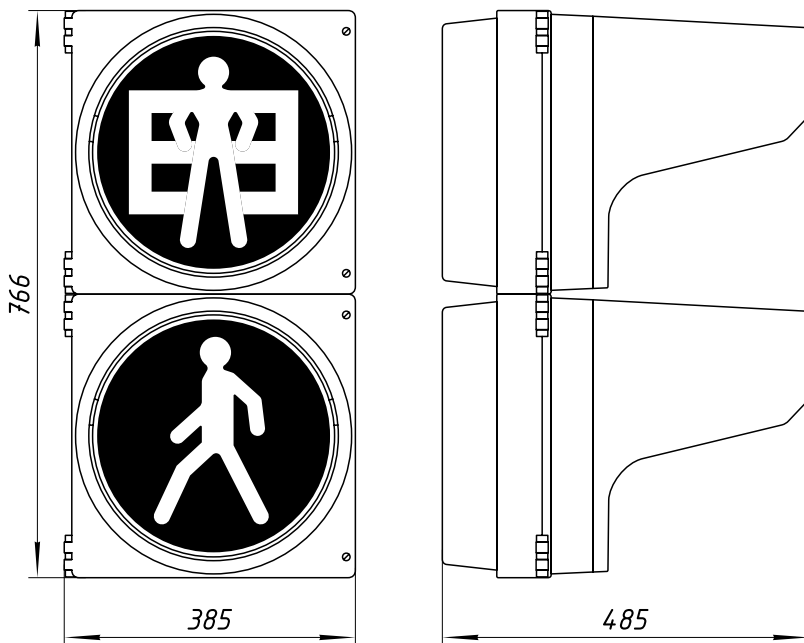
Рис. 1. Общий вид и габаритные размеры пешеходного светофора с обратным отсчетом времени с диаметром выходной апертуры 300 мм
