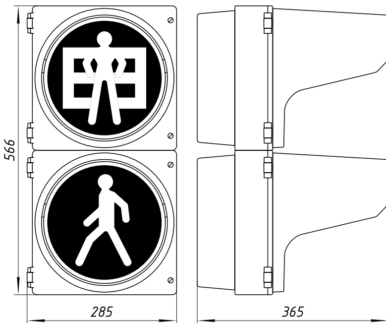
Рис. 1. Общий вид и габаритные размеры пешеходного светофора с обратным отсчетом времени с диаметром выходной апертуры 200 мм
