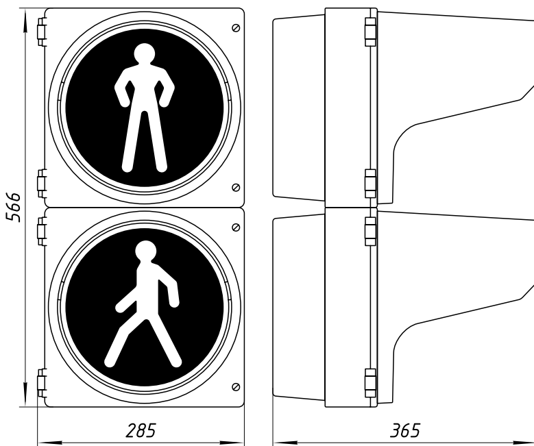
Рис. 1. Общий вид и габаритные размеры пешеходного светофора с диаметром выходной апертуры 200 мм
