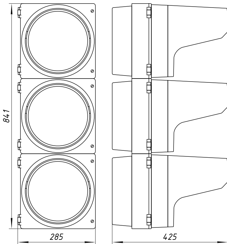
Рис. 1. Общий вид и габаритные размеры светофора
