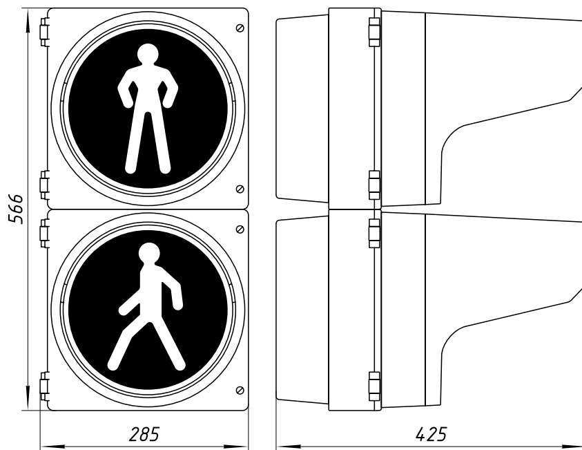
Рис. 1. Общий вид и габаритные размеры пешеходного лампового светофора с диаметром выходной апертуры 200 мм
